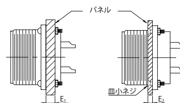
前面取付け
