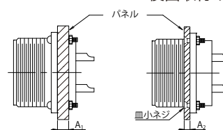
前面取付け
